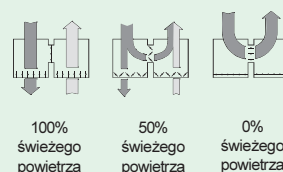
Schemat funkcji mieszania
