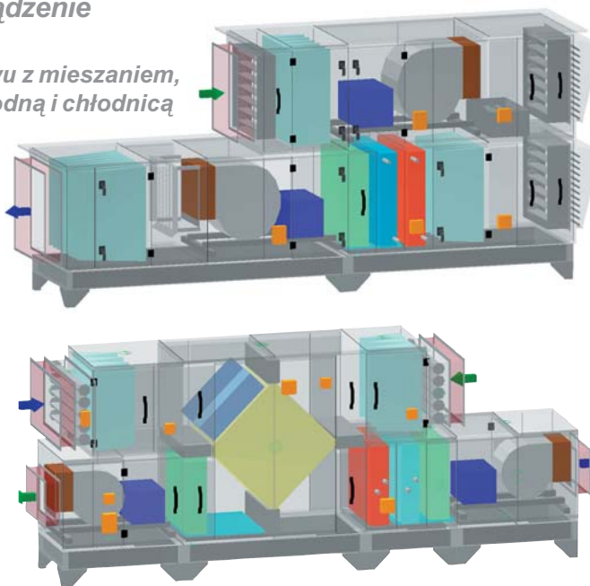
przykład zestawu z rekuperatorem krzyżowym, z nagrzewnicą wodną i chłodnicą
