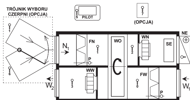
widok z przodu / wykonanie centrali „prawe” (RO-KPE)
