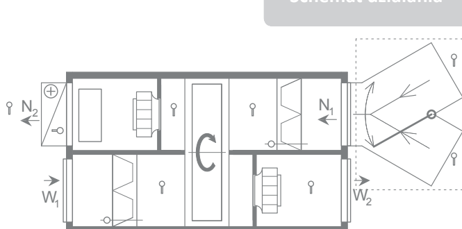
widok z przodu / wykonanie centrali „lewe” (RO-KPEL)
