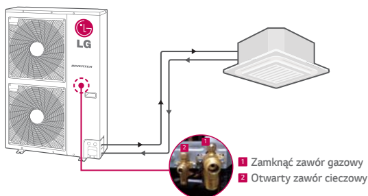
Wypompowywanie czynnika chłodniczego*
